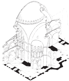
aksonometrik izdüşüm
